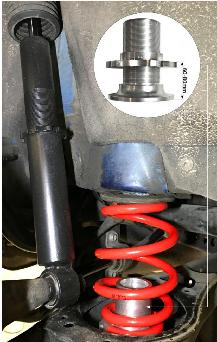
Fahrwerk Achse 2
